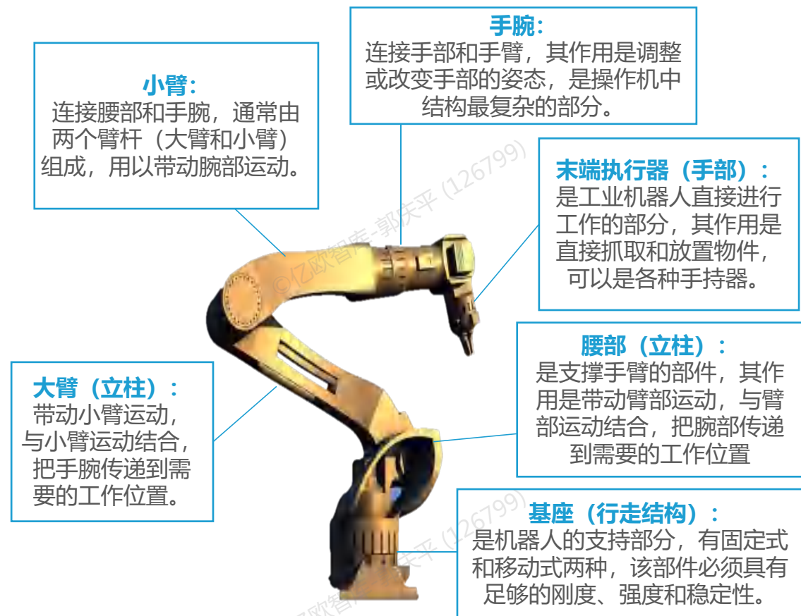
亿欧智库：工业机器人机械结构
