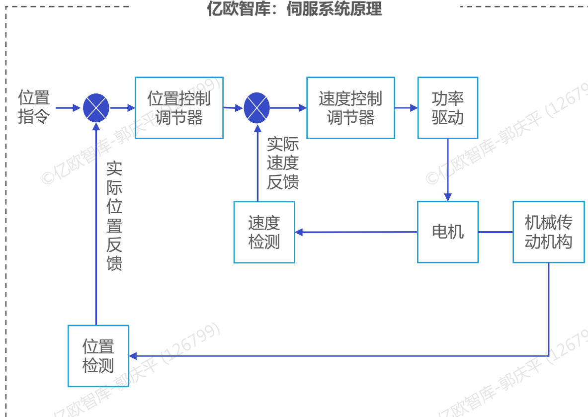
亿欧智库：伺服系统原理
