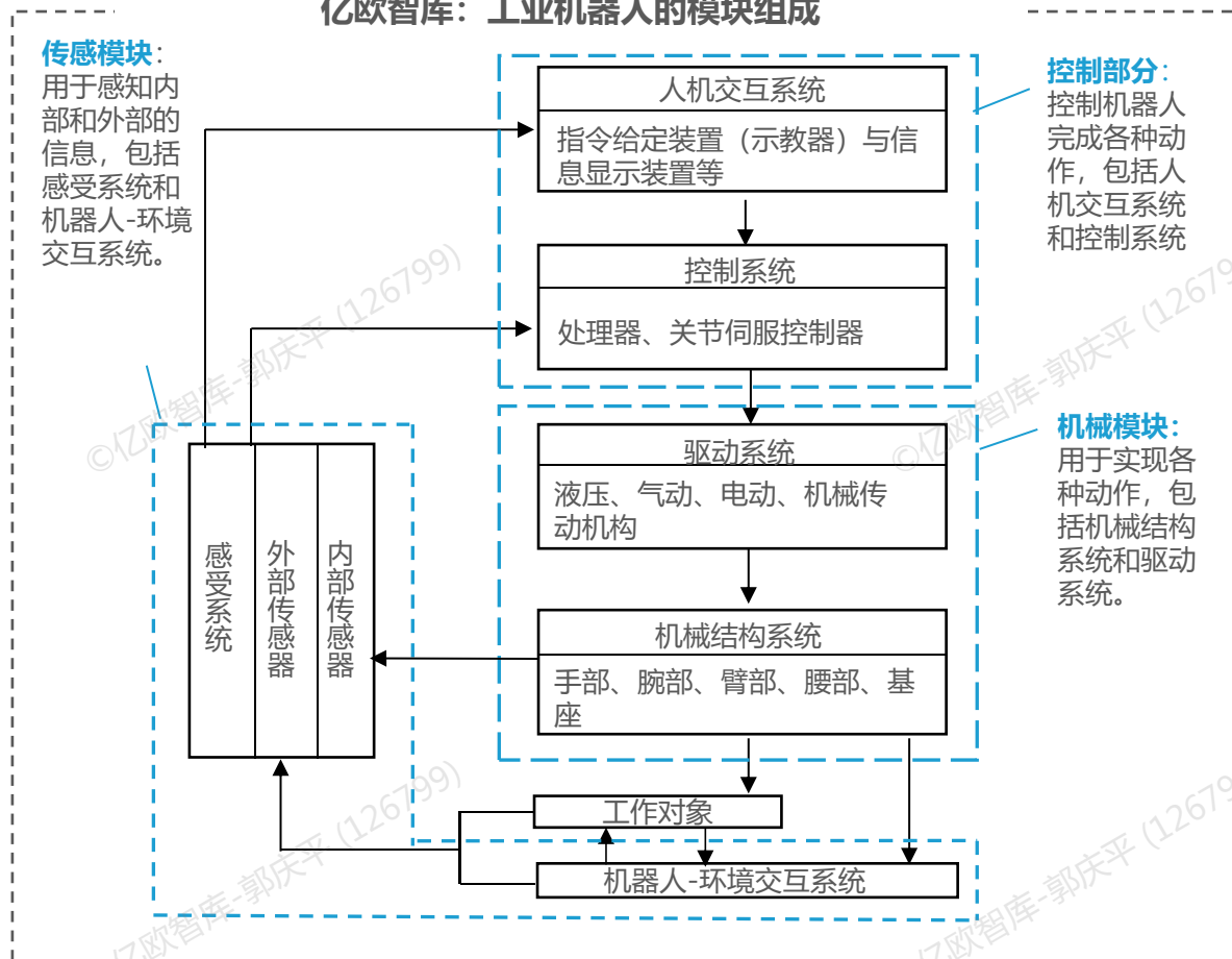
亿欧智库：工业机器人的模块组成
