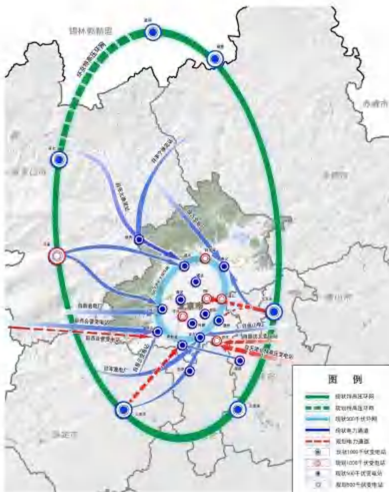
图 4 2025 年北京电网规划布局示意图
